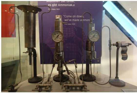
Procédé Haber de synthèse de l'ammoniac
